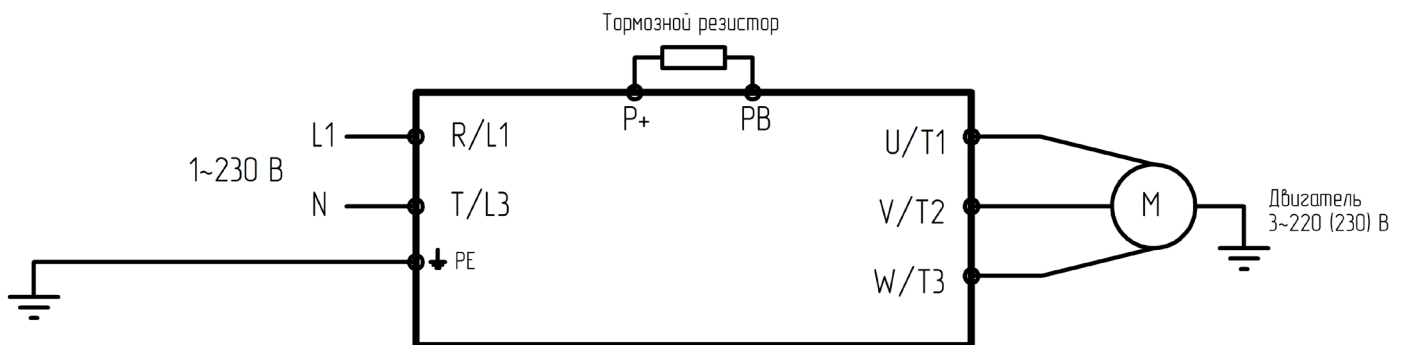
Подключение силовых клемм для моделей LCI-GY/PY-2(B)
