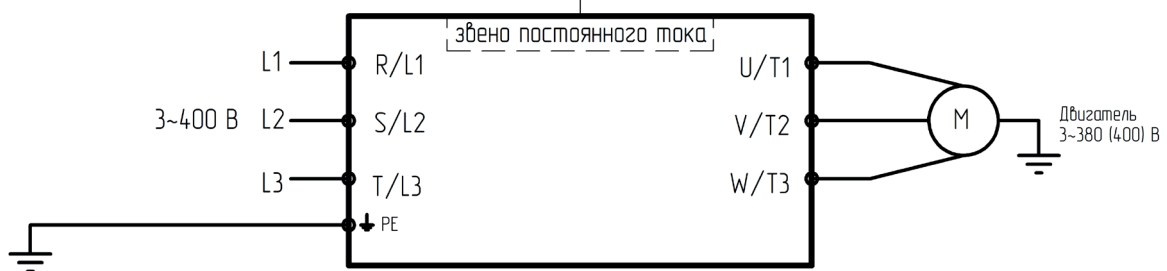
Подключение силовых клемм для моделей LCI-GY/PY-4(B)
