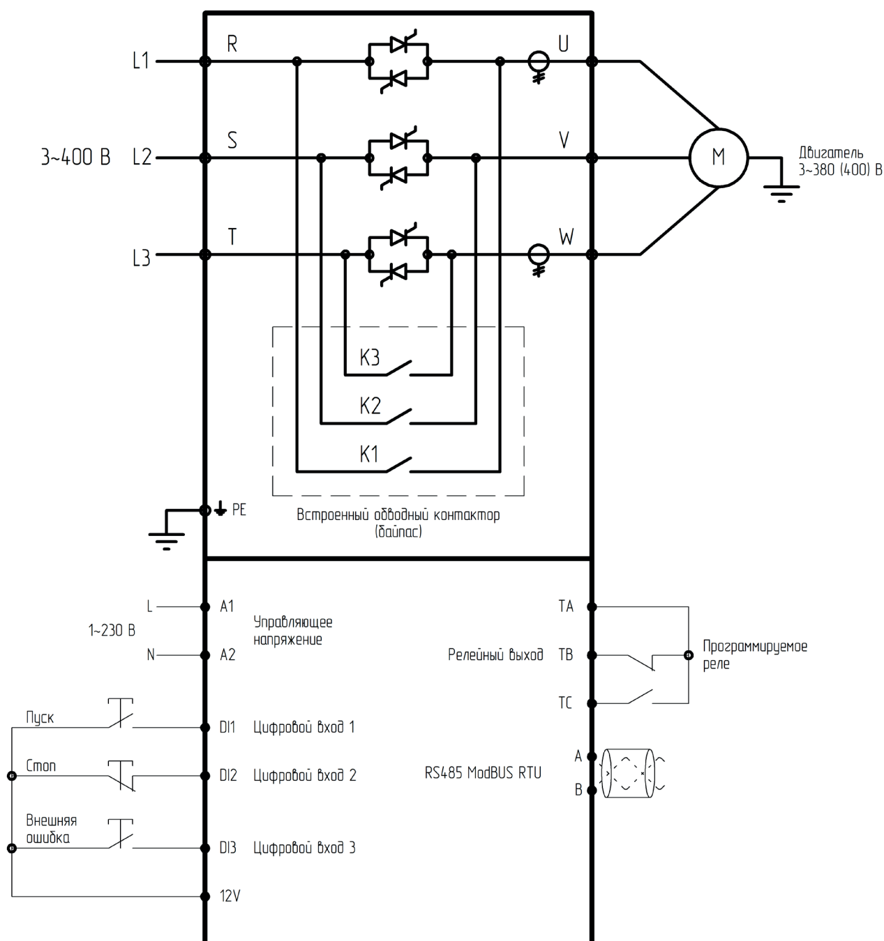
Стандартная конфигурация УПП SBIM мощностью до 15 кВт
