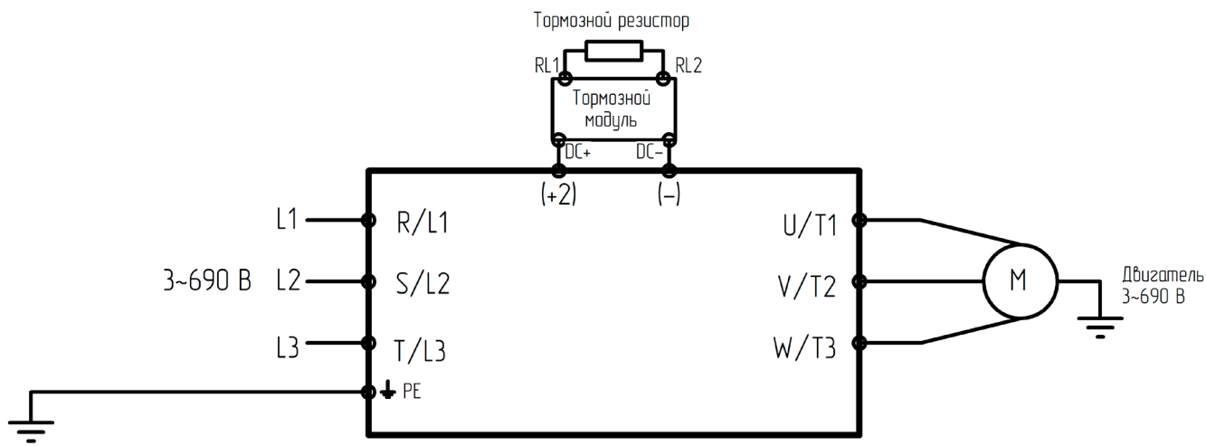
Подключение силовых клемм для моделей LCI-GY/PY-6
