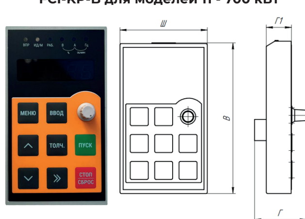
FCI-KP-B для моделей 11 - 700 кВт
